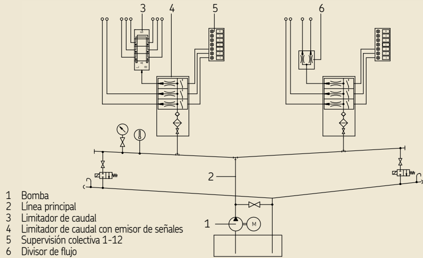
Ejemplo de un sistema de lubricación por circulación de aceite
